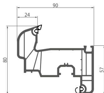
047 Стулка 6-камерна
