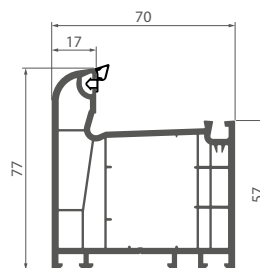
082 Дверна рама
