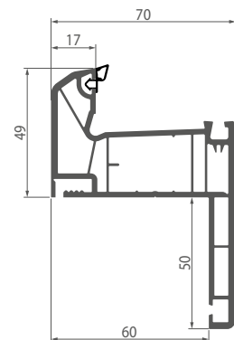
081 Реноваційна рама
