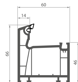
001 Рама 4-камерна
