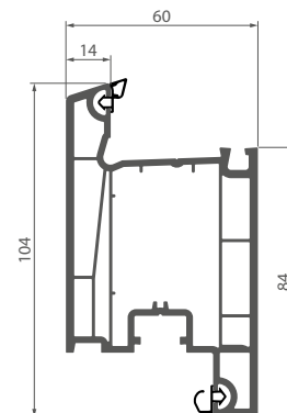
056 Дверна стулка зовнішнього відкривання
