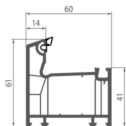
086 Рама 5-камерна
