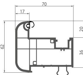
054 Штульп
