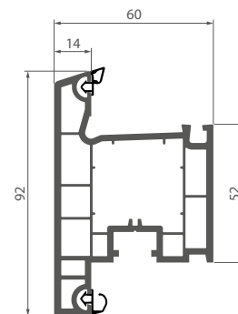
056 Дверна стулка зовнішнього відкривання
