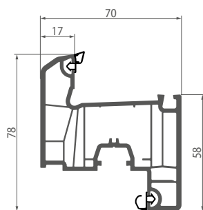
081 Реноваційна рама
