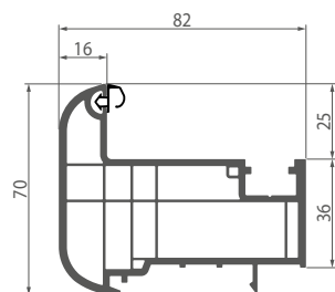
068 Штульп
