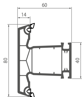
027 Імпост 4-камерний
