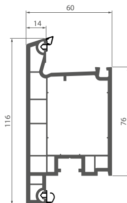
036 Дверна стулка зовнішнього відкривання
