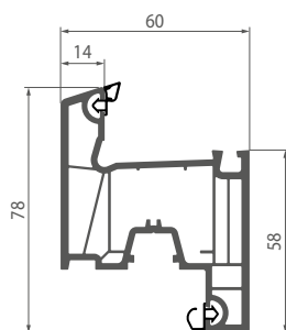
087 Стулка 5-камерна
