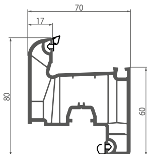
060 Стулка 6-камерна
