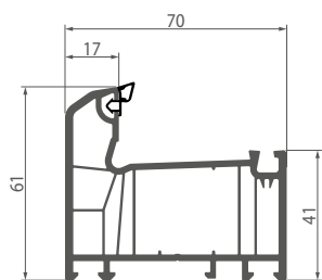
088 Рама 6-камерна
