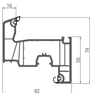
068 Штульп
