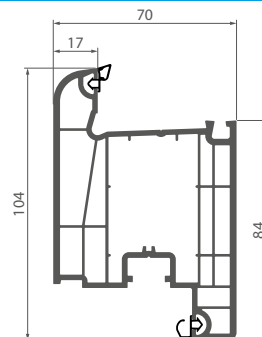
078 Дверна стулка внутрішнього відкривання
