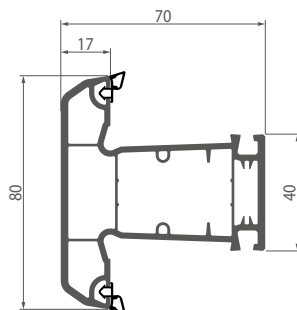
054 Штульп
