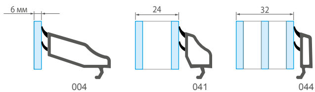
Штапики
