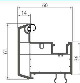
012 Штульп
