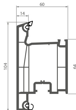
036 Дверна стулка зовнішнього відкривання
