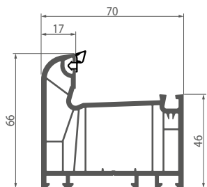
092 Рама 6-камерна Class A
