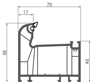
059 Рама 6-камерна
